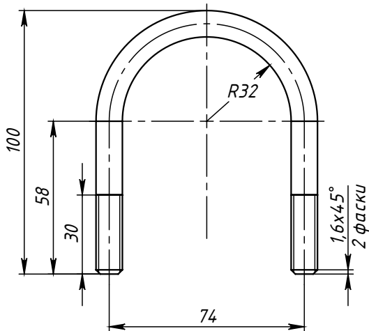
Поз.5 (Хомут)
