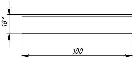
Поз.3 (Ложемент)
